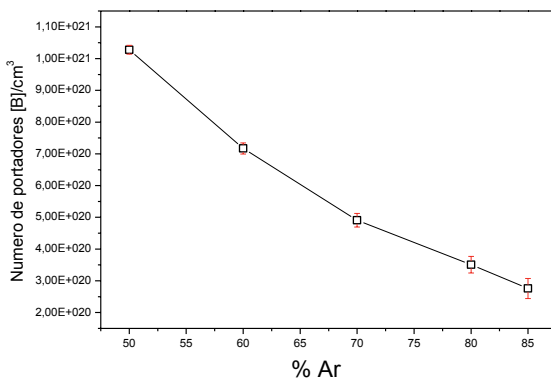
Figura 5.5 - Gráfico mostrando o número de portadores de boro obtidos pela equação 3.5 por variações da concentração de argônio com as respectivas barras de erro.
