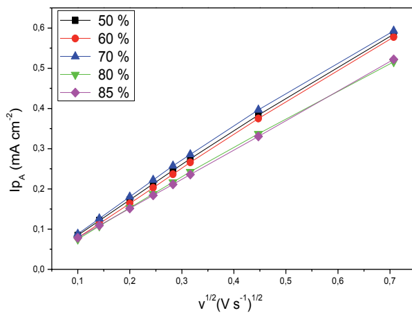
Figura 5.12 - Corrente de oxidação ( I_p ) por raiz quadrada da velocidade de varredura por variações da concentração de argônio.
