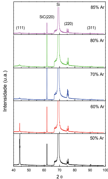
Figura 5.6 - Difratogramas de raios-X mostrando os planos cristalográficos (111), (220) e (311) do diamante, além do sinal do silício e do carbeto de silício SiC, em função da concentração de argônio.
