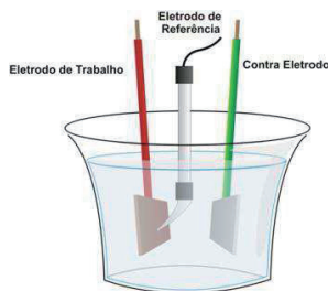
Figura 3.6 – Célula eletroquímica de três eletrodos
