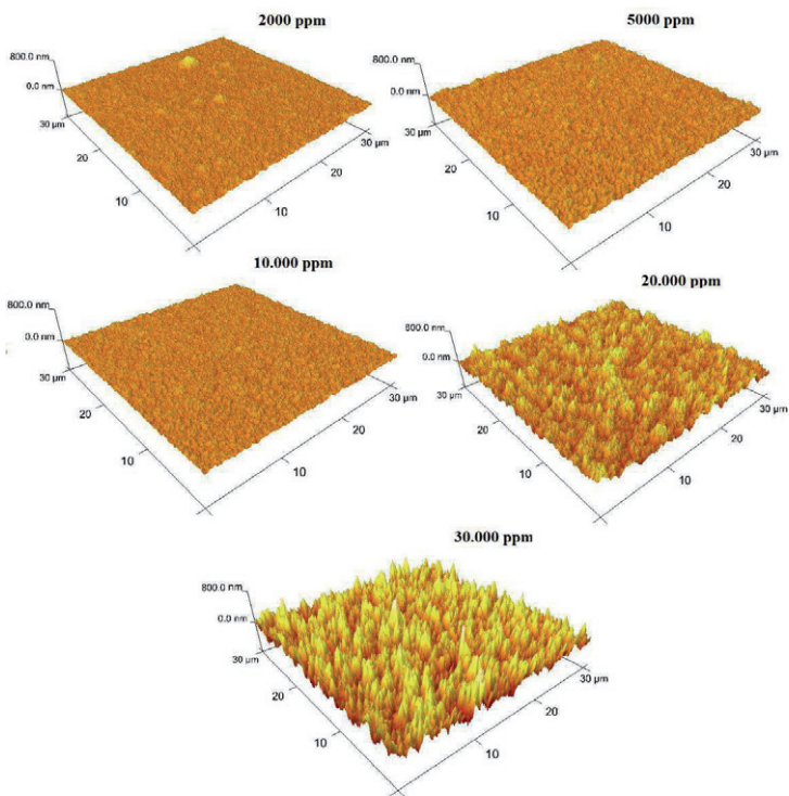
Figura 4.7 - Imagens obtidas por MFA dos filmes de diamante em diferentes níveis de dopagem em um tempo de crescimento de 16 h.
