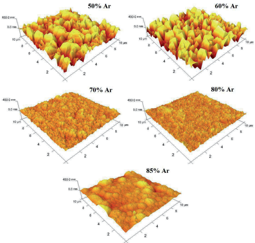
Figura 5.3 - Imagens MFA das amostras por variações da concentração de argônio.
