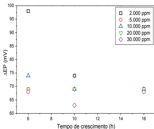
Figura 4.19 - Variação do potencial de pico ( \Delta E_p = E_{pC} - E_{pA} ) em velocidade de varredura de 100 mv/s para eletrodos com diferentes níveis de dopagem e tempos de crescimento.
