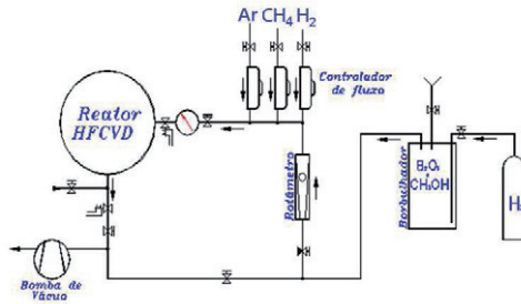
Figura 3.3 - Configuração externa do reator de filamento quente.
