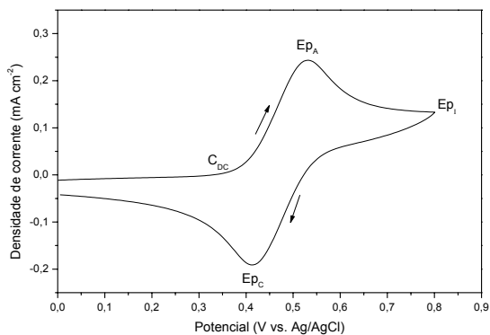
Figura 3.7 - Exemplo da curva do sistema redox em ferrocianeto ( (\text{Fe}(\text{CN})_6)^{-3/4} ) obtidas por Voltametria Cíclica para uma velocidade de varredura de 100 mV/s para um filme DUNDB deste trabalho (2.000 ppm e 6 h). A seta indica o sentido de varredura, e as marcações identificam os potenciais de pico anódico ( E_{pA} ), de inversão ( E_{pI} ) e catódico ( E_{pC} ), além de identificar o trecho de carregamento da dupla camada ( C_{DC} ).
