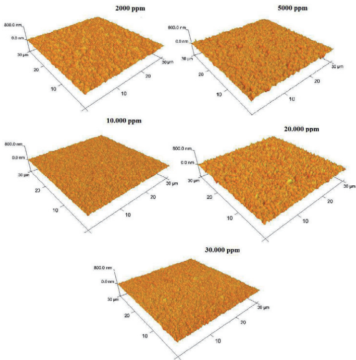
Figura 4.6 - Imagens obtidas por MFA dos filmes de diamante em diferentes níveis de dopagem em um tempo de crescimento de 10 h.
