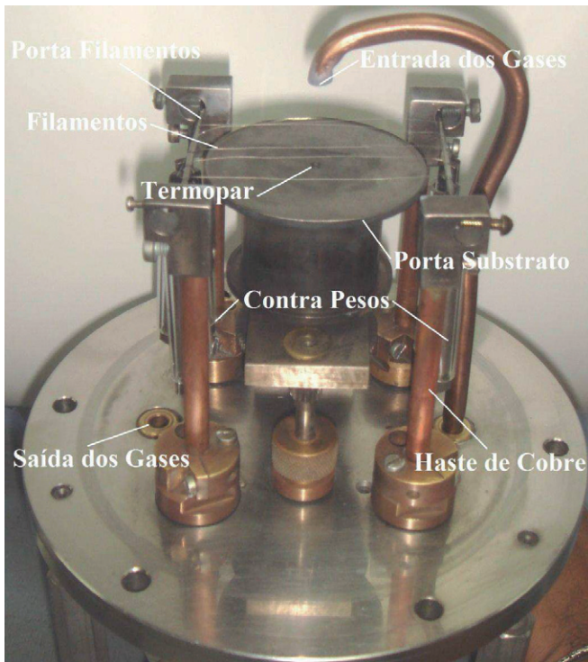
Figura 3.2 - Imagem interna do reator de filamento quente.
