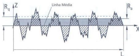
Figura 3.4 - Esquema de uma superfície rugosa mostrando a linha média e as rugosidades média (Ra) e média quadrática (Rq).
